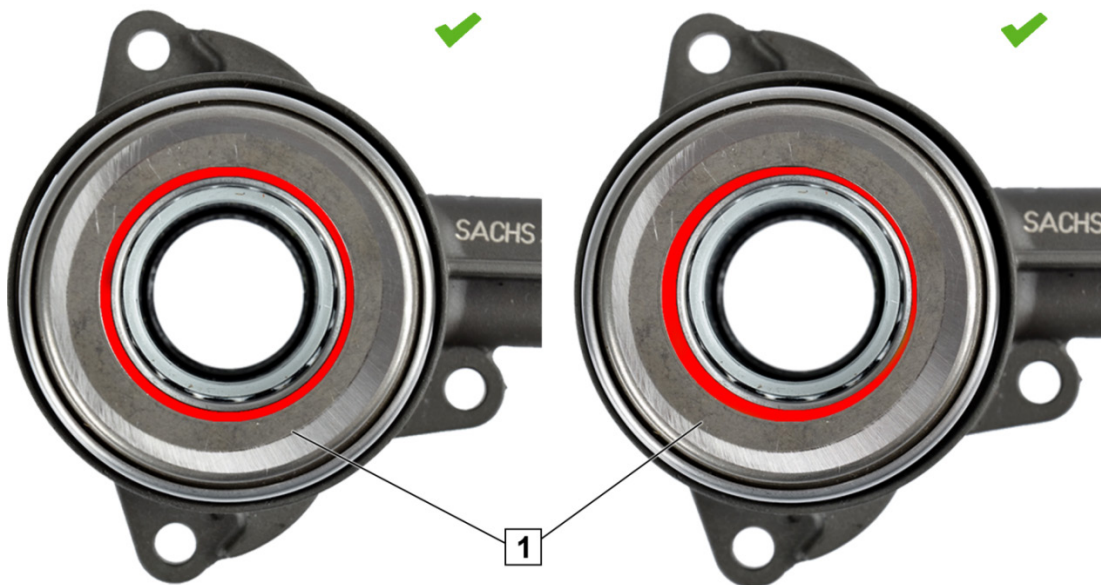
Afb. 2: CSC met zelfcentrering. Lager gecentreerd en niet-gecentreerd (voorbeeld).
