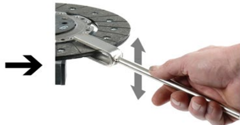
Afb. 4: Koppelingsplaat rechtzetten
