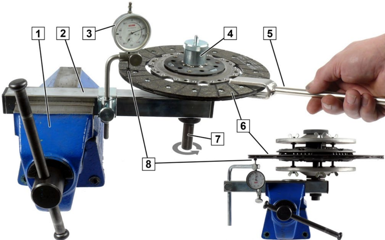
Afb. 1: Testapparaat voor uitsparing aan de zijkant Pkw
