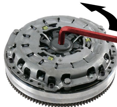
Fig. 3 : Retirer la pièce de verrouillage en tournant
