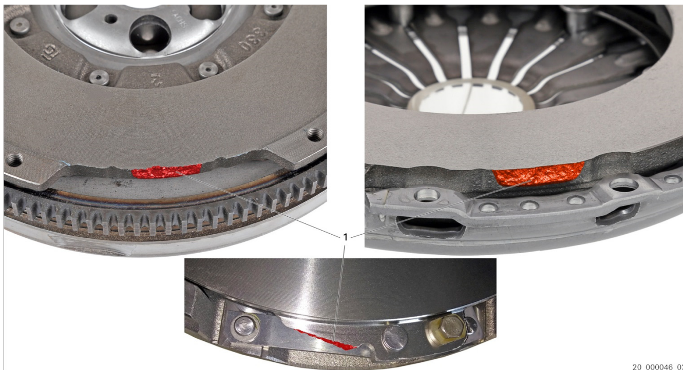
Fig. 1: canto de rotura (ejemplo)
