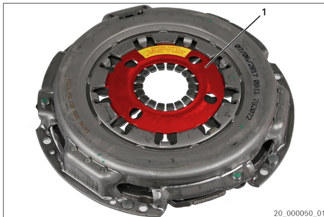
Fig. 5: XTend Tipo III con pieza de bloqueo
