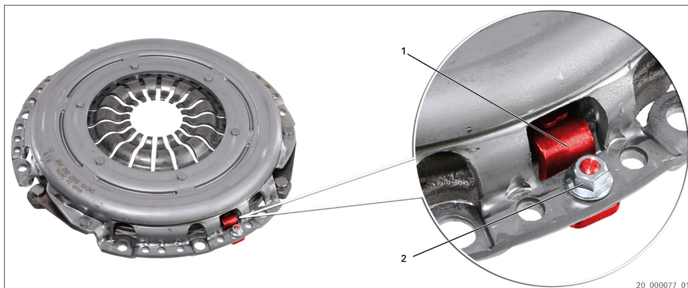
Fig. 2: XTend Tipo I con tope de la carcasa (atornillado)
