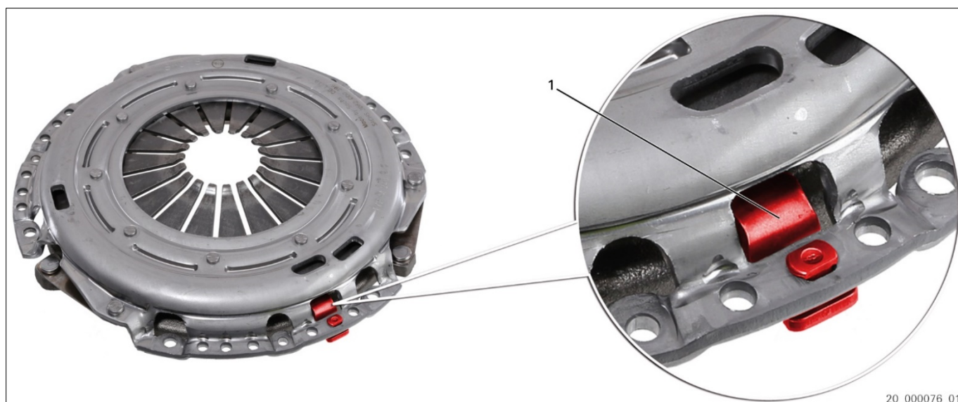
Fig. 1: XTend Tipo I con tope de la carcasa (remachado)
