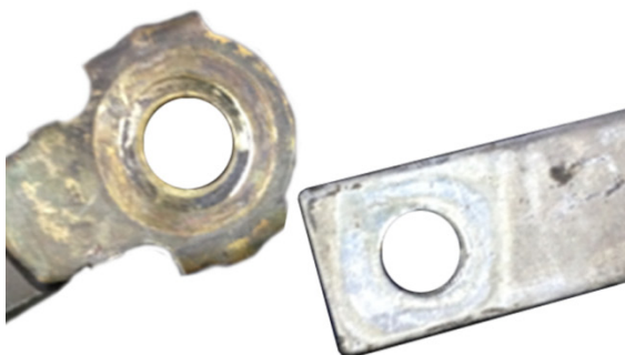
Abb. 1: Masseverbindung vor der Reinigung: Kontakt schlecht
