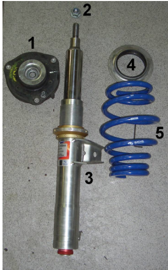
Vorderachse
